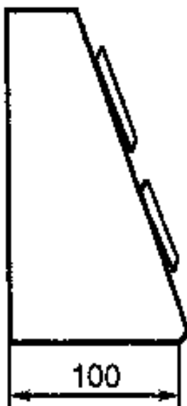
Рисунок G.1. Пример управления XL устройства в кабине лифта (вид сбоку)
